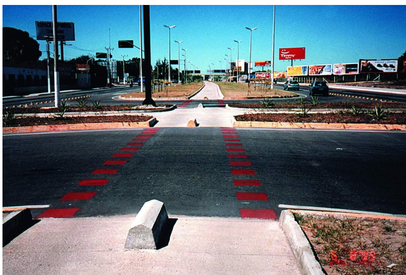
FIGURA 107 TRAVESSIA DA CICLOVIA DA AV. WASHINGTON SOARES
